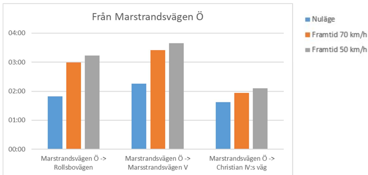
Figur 41 Restider från Marstrandsvägen Ö
