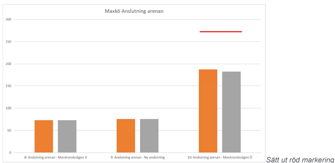
Figur 27 Maxkö vid ny anslutning till Arenan. Staplarna visar Marstrandsvägen V, ny anslutning och Marstrandsvägen Ö.
