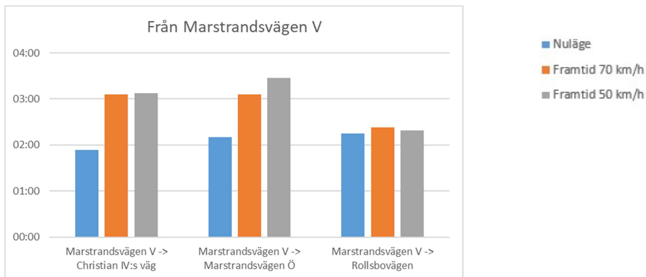
Figur 35 Restider från Marstrandsvägen V.
