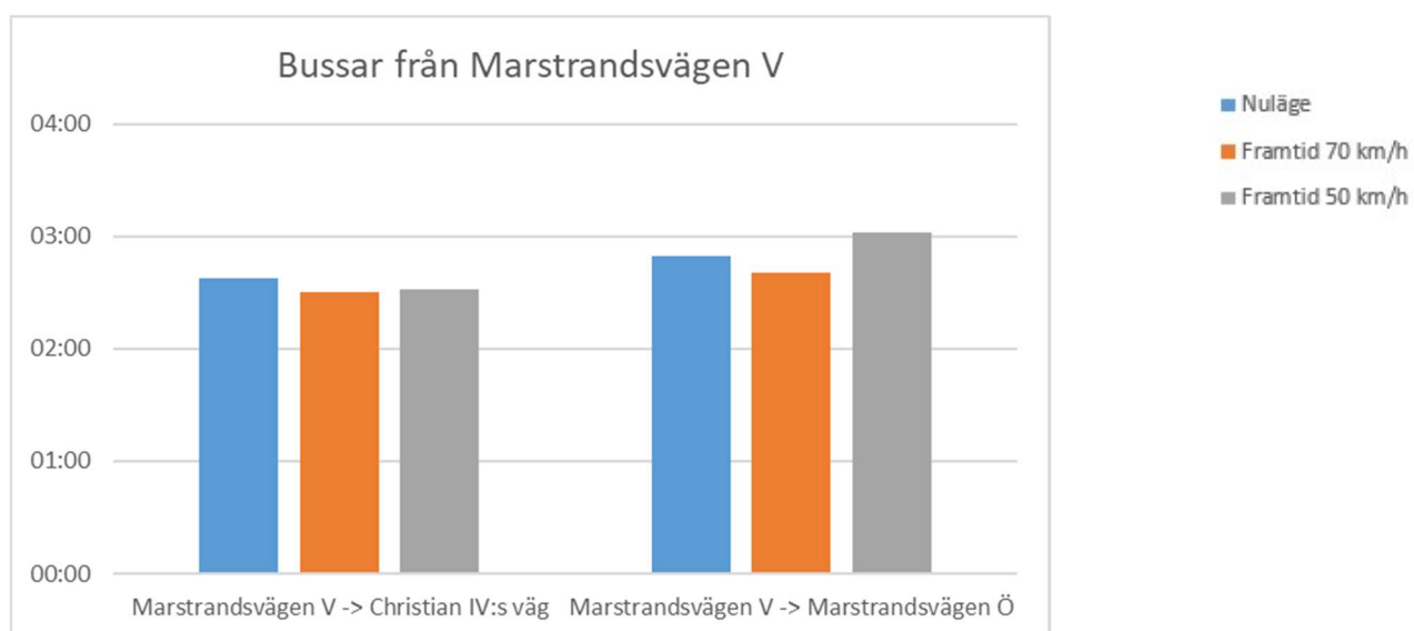
Figur 36 Bussarnas restider från Marstrandsvägen V
