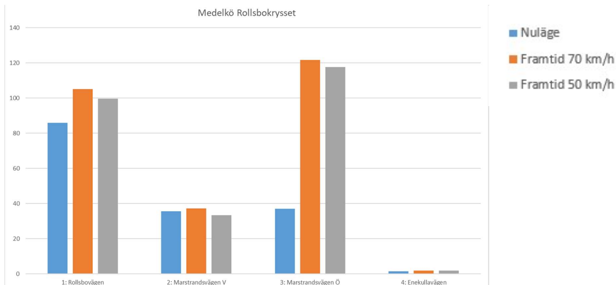
Figur 28 Medelkö vid Rollsbovägen. Staplarna visar Rollsbovägen, Marstrandsvägen V, Marstrandsvägen Ö och Enekullsvägen.
