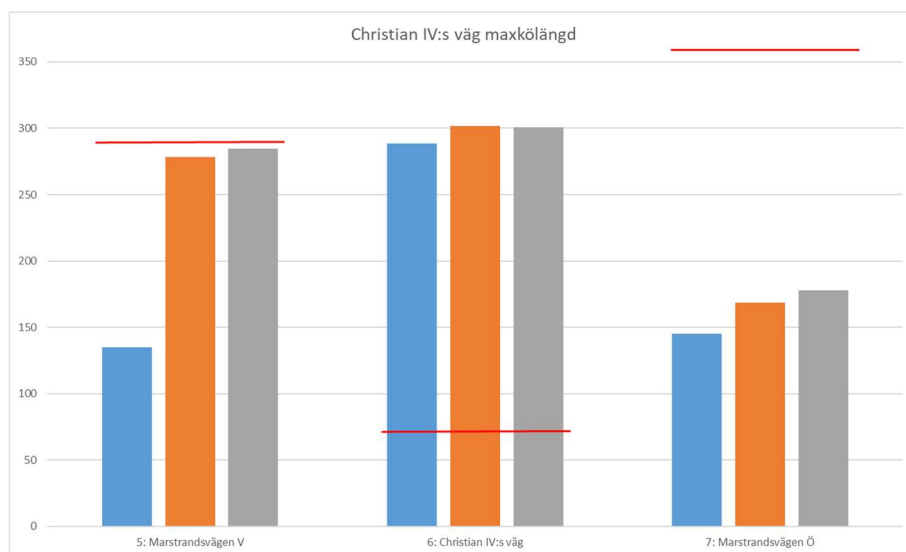
Figur 31 Maxkö vid Christian IV:s väg. Staplarna visar Marstrandsvägen V, Christian IV:s väg och Marstrandsvägen Ö.
