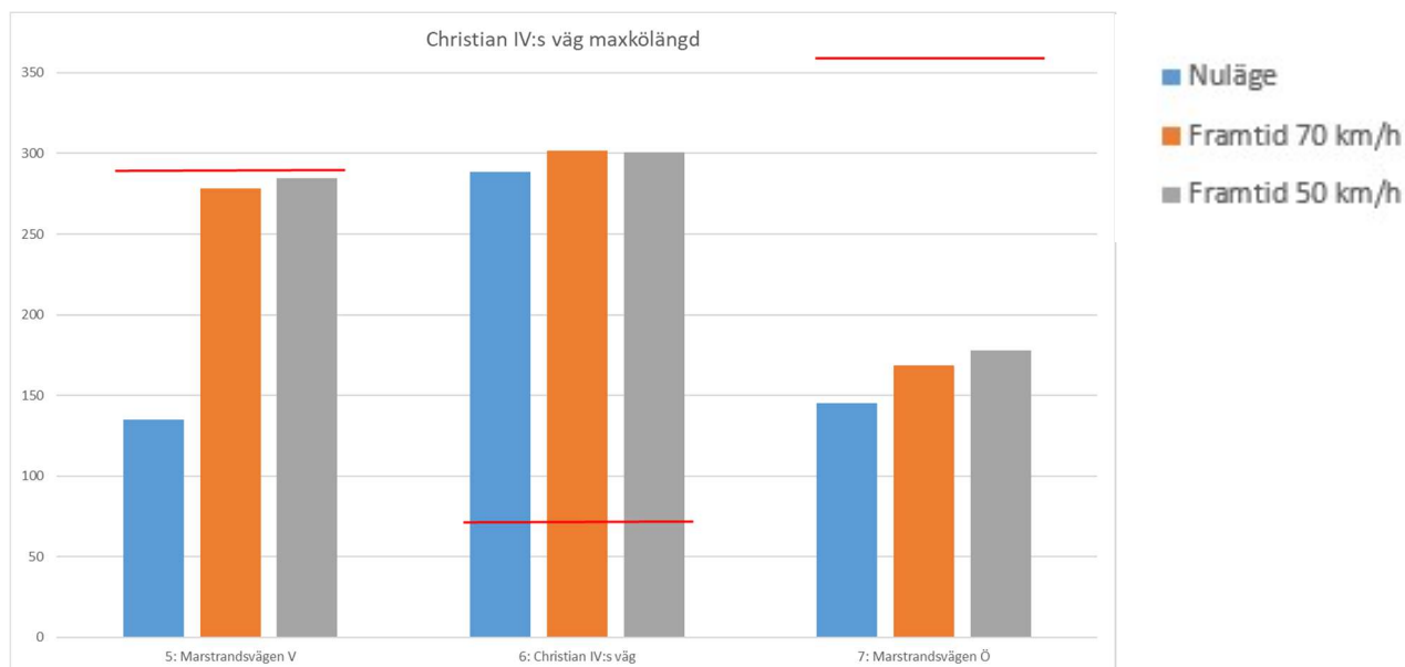
Figur 18 Maxkö i meter vid Christian IV:s väg. Röd linje visar avstånd till nästa korsning. Staplarna visar Marstrandsvägen V, Christian IV:s väg och Marstrandsvägen Ö.
