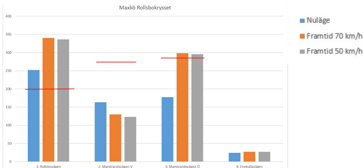
Figur 29 Maxkö vid Rollsbovägen. Staplarna visar Rollsbovägen, Marstrandsvägen V, Marstrandsvägen Ö och Enekullsvägen.
