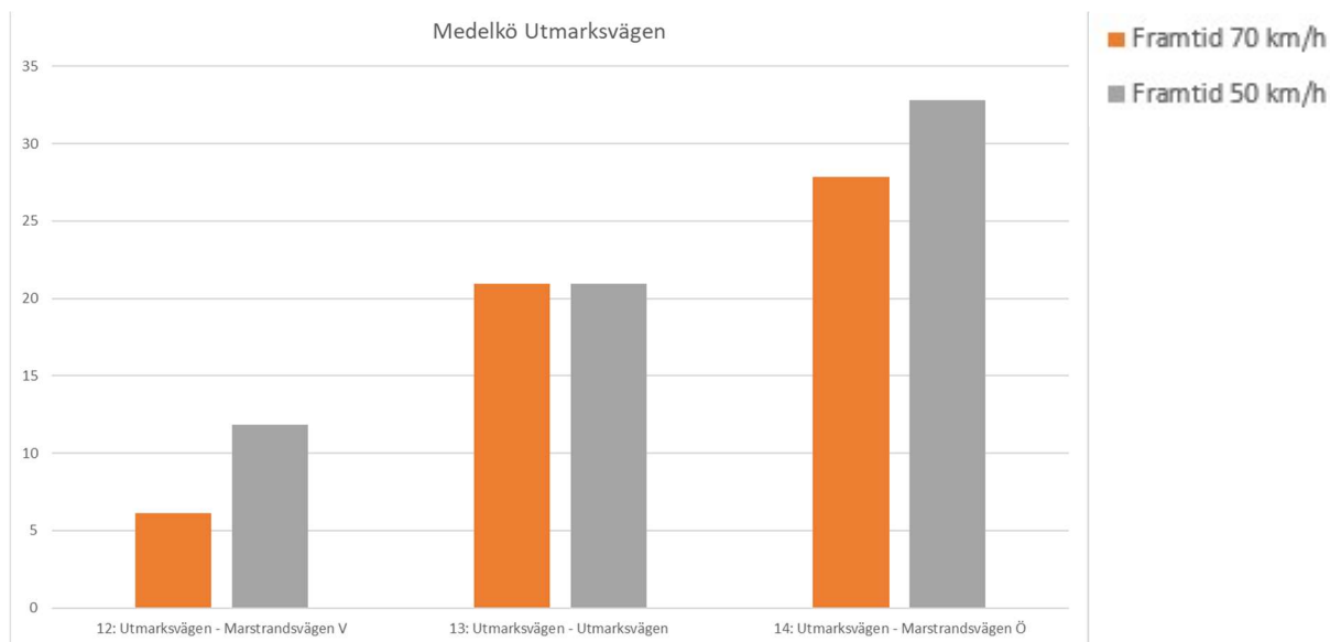
Figur 32 Medelkö vid ny anslutning till Åseberget via Utmarksvägen. Staplarna visar Marstrandsvägen V, ny anslutning och Marstrandsvägen Ö.
