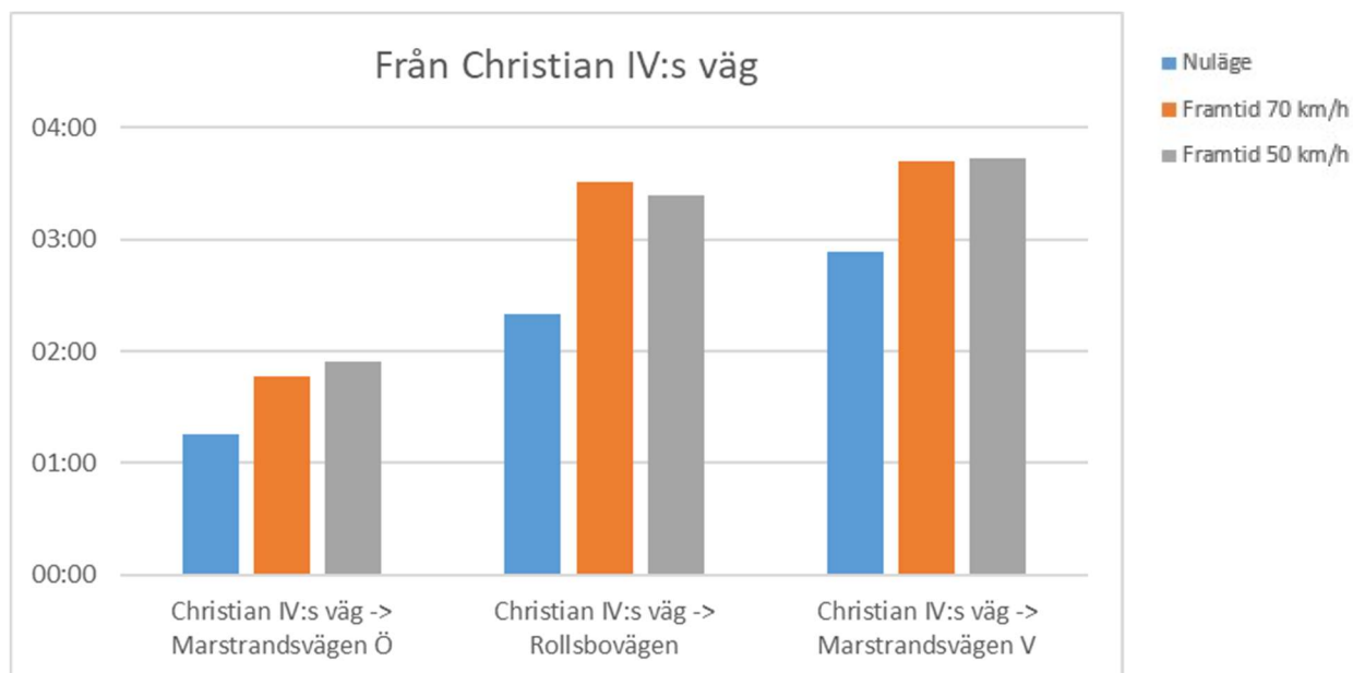
Figur 38 Restider från Christian IV:s väg.
