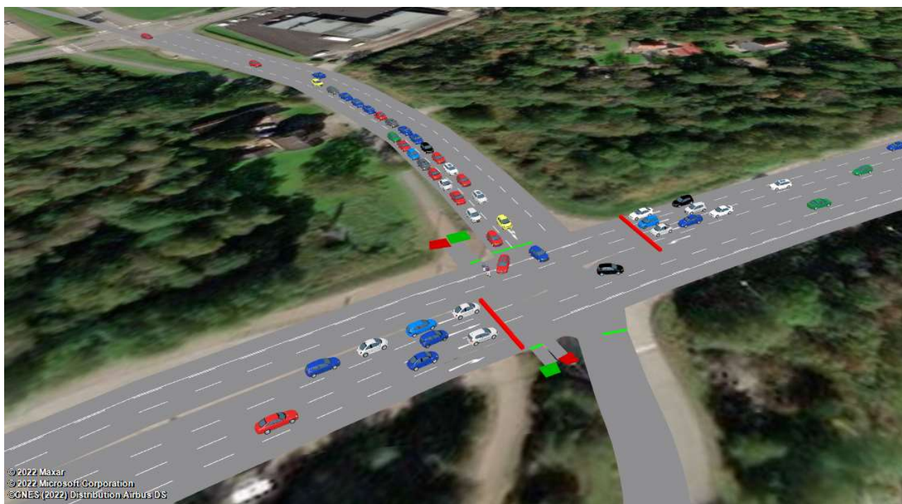
Figur 25 Högersvängande fordon som åker ut på Marstrandsvägen från Rollsbovägen får vänta på personer som korsar övergångsstället trots att motorfordon har grönt ljus.
