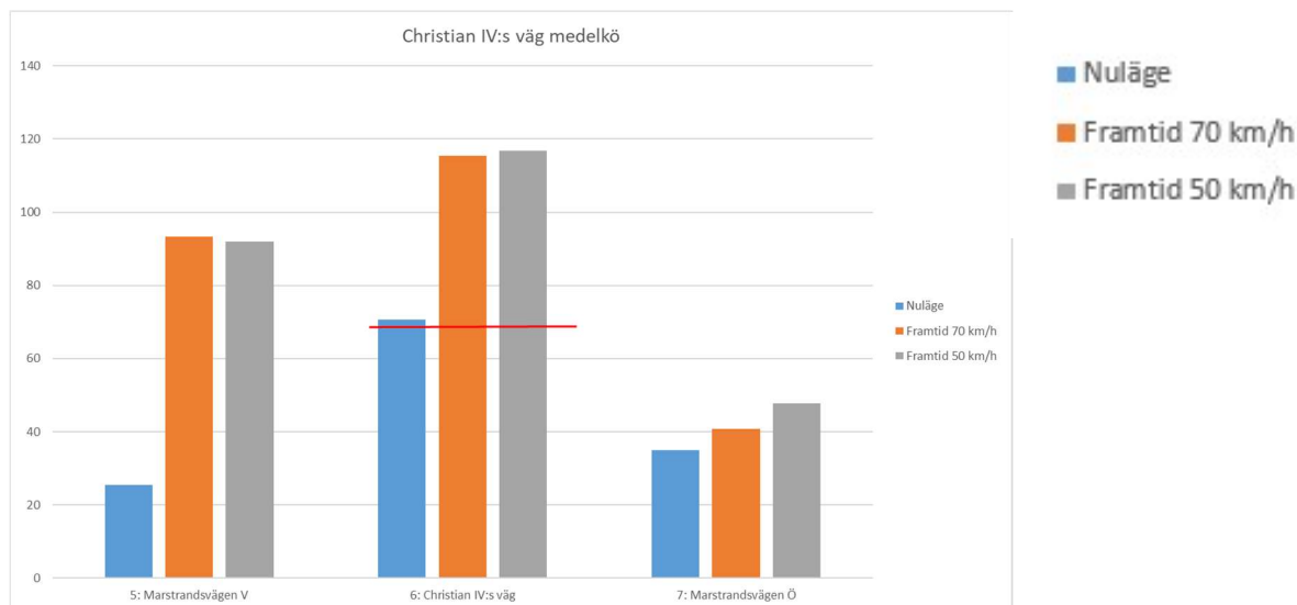
Figur 30 Medelkö vid Christian IV:s väg. Staplarna visar Marstrandsvägen V, Christian IV:s väg och Marstrandsvägen Ö.
