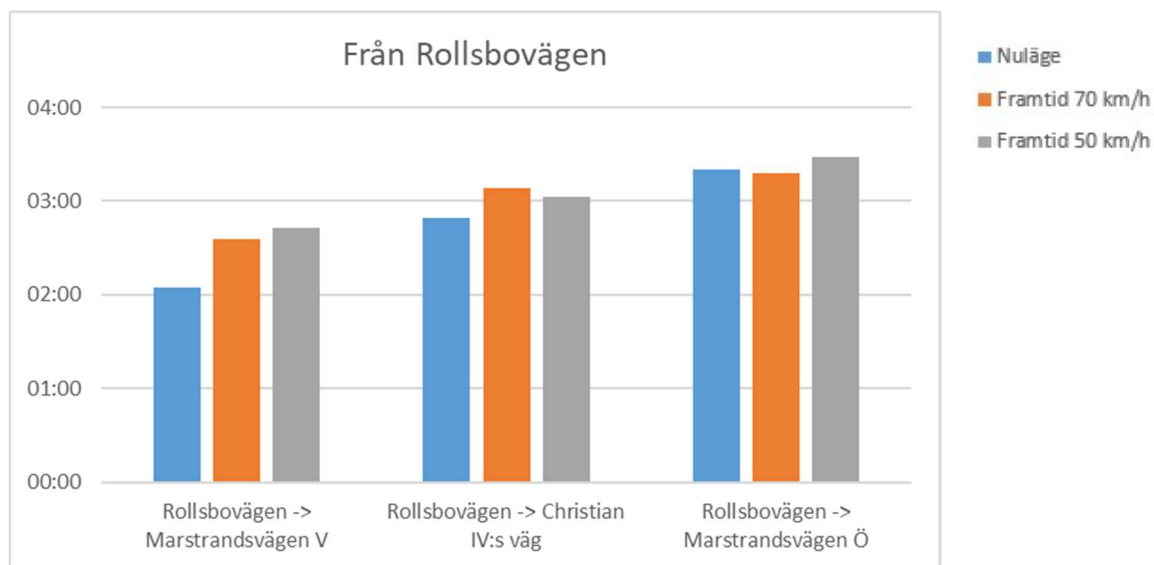
Figur 44 Restider från Rollsbovägen
