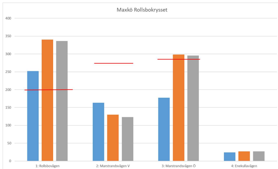
Figur 16. Maxkö i meter vid Rollsbokrysset. Röd linje visar avstånd till nästa korsning. Staplarna visar Rollsbovägen, Marstrandsvägen V, Marstrandsvägen Ö och Enekullavägen.
