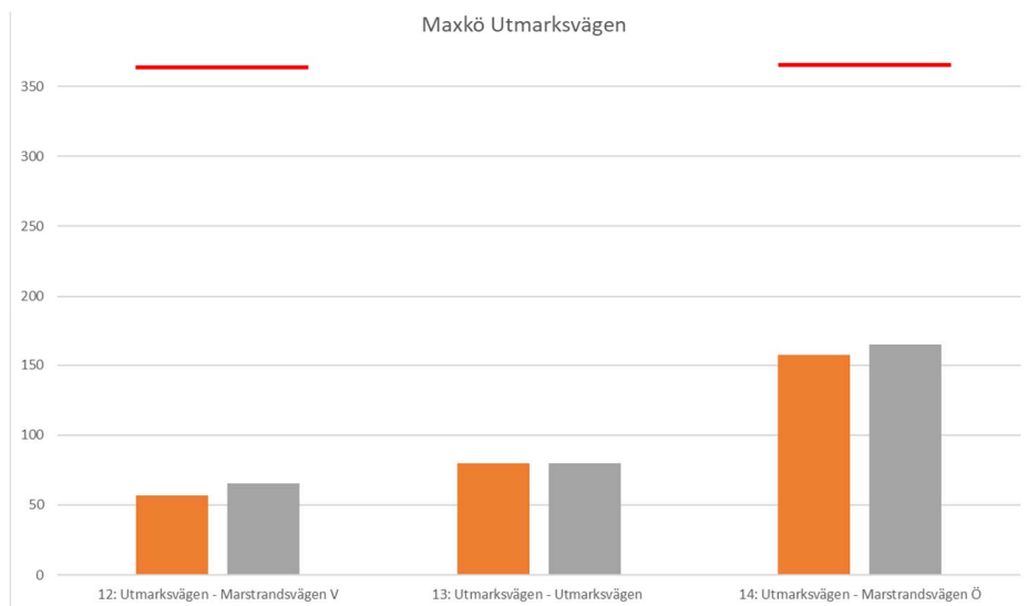
Figur 20 Maxkö vid ny anslutning till Åseberget, via Utmarksvägen. Staplarna visar Marstrandsvägen V, ny anslutning och Marstrandsvägen Ö.
