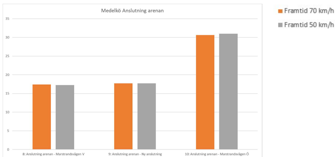
Figur 26 Medelkö vid ny anslutning till Arenan. Staplarna visar Marstrandsvägen V, ny anslutning och Marstrandsvägen Ö.
