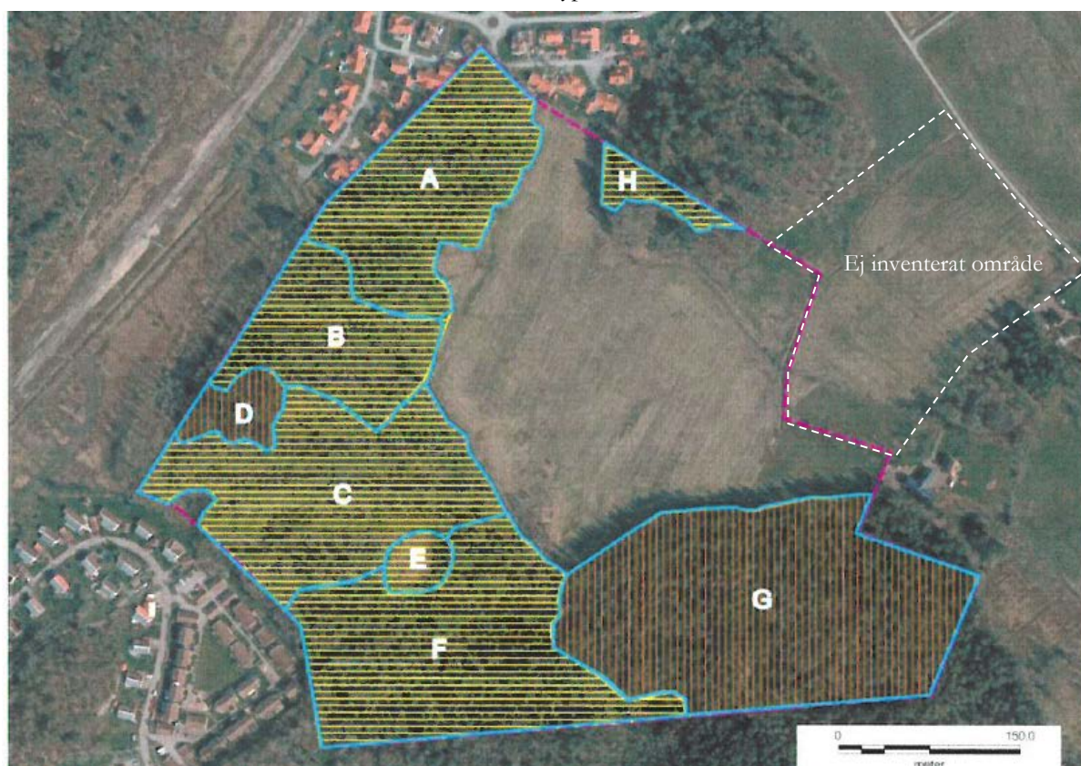
Bild 10: Naturvärdesklassning (Norconsult, 2015)
