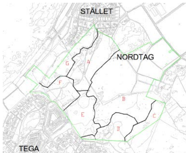
Bild 27; Avrinningsområden (SWECO, 2016)
