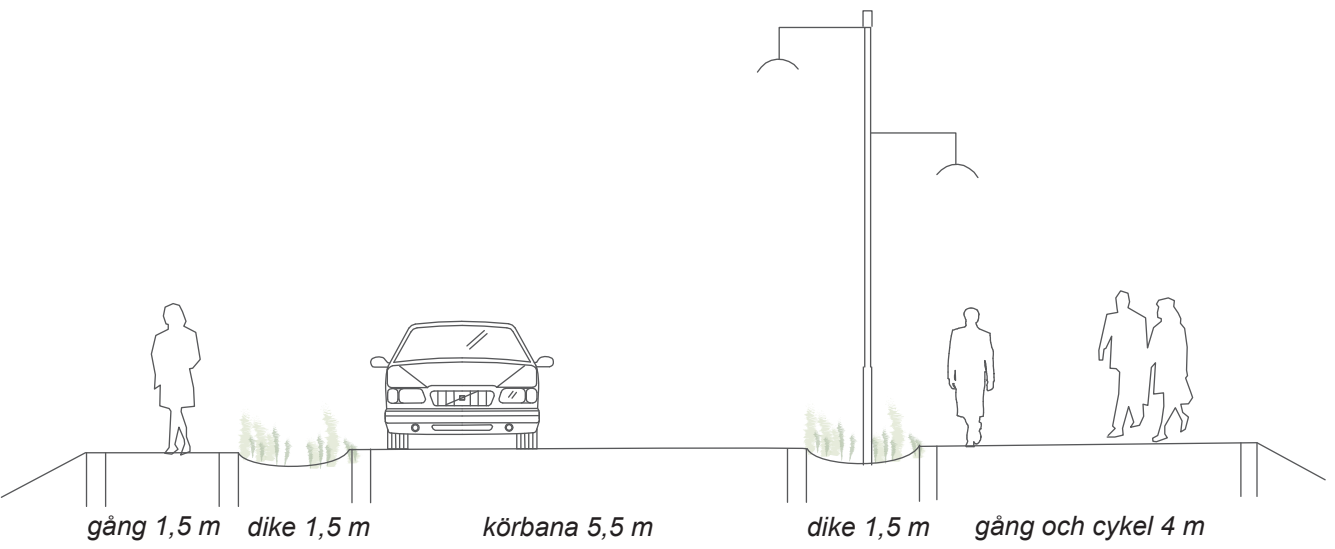
Gata 1 (sektion B-B) : Vägbredd 15 m
