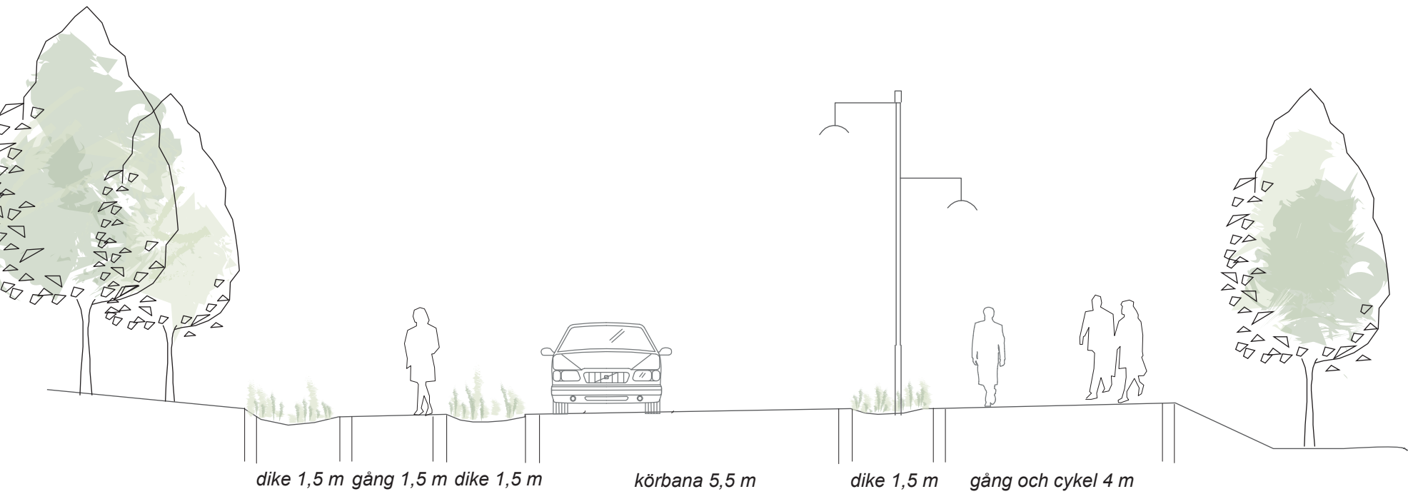
Gata 1 (sektion A-A) : Vägbredd 17 m
