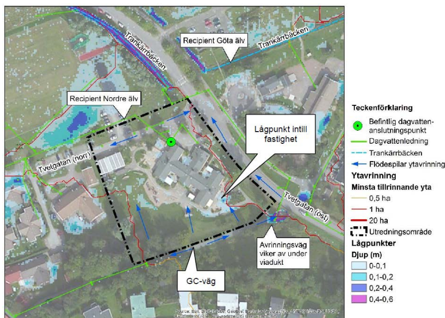
Bild 7, Befintlig dagvattenavledning samt ytavrinningsvägar och lågpunkter i händelse av ett kraftigt regn då ledningsnätet går fullt (OBS: Höjdmödel RH 2000).
