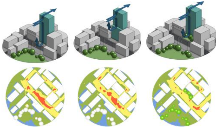
Figur 7. Effekten av en hög byggnad på vinden i gaturummet. Den övre bilden visar byggnadsutformning, och vindflöde (blå pilar). De undre bilderna representerar ytor med vindhastigheter över vissa tröskelvärden, där grönt representerar mindre blåsiga områden och rött visar mer blåsiga områden. Bild modifierad från Lynch (2023).
