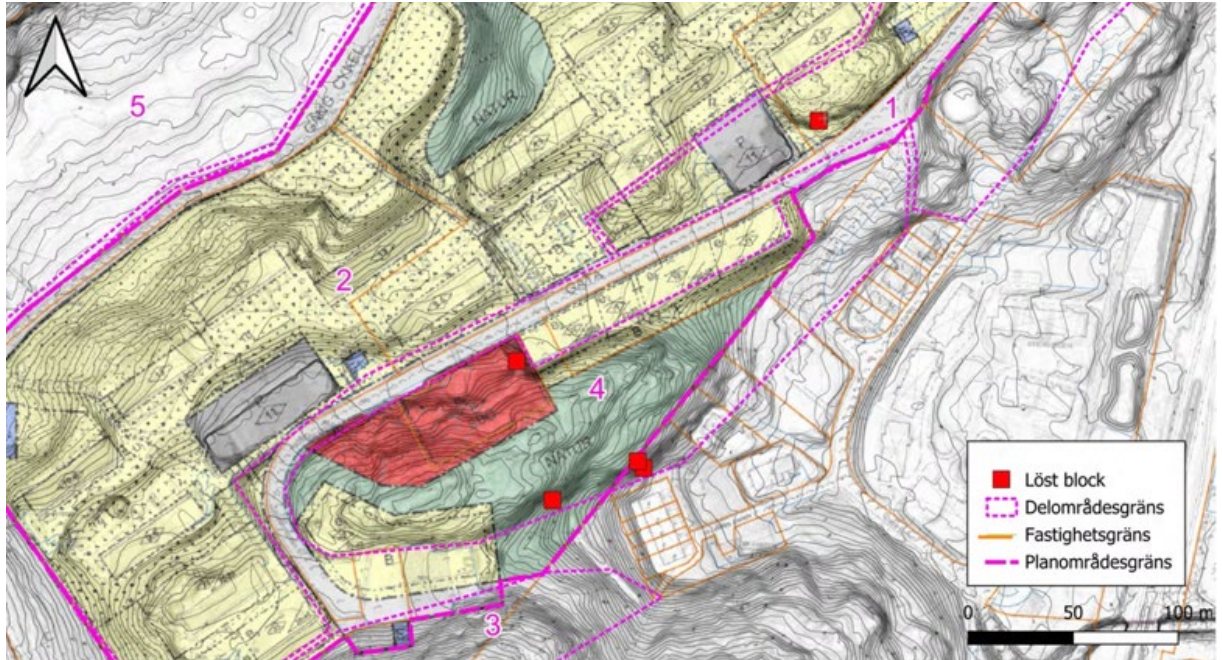
Figur 11. Löst sittande block, lokaliserade under bergteknisk utredning.
